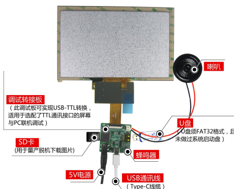
图 1-4 调试工具图
